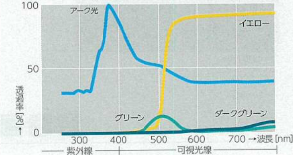
全光線透過率グラフ
