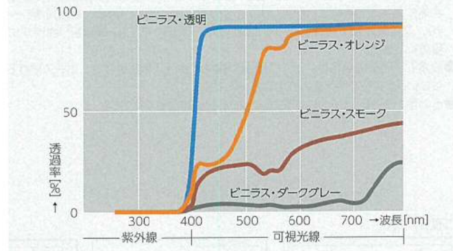
全光線透過率グラフ
